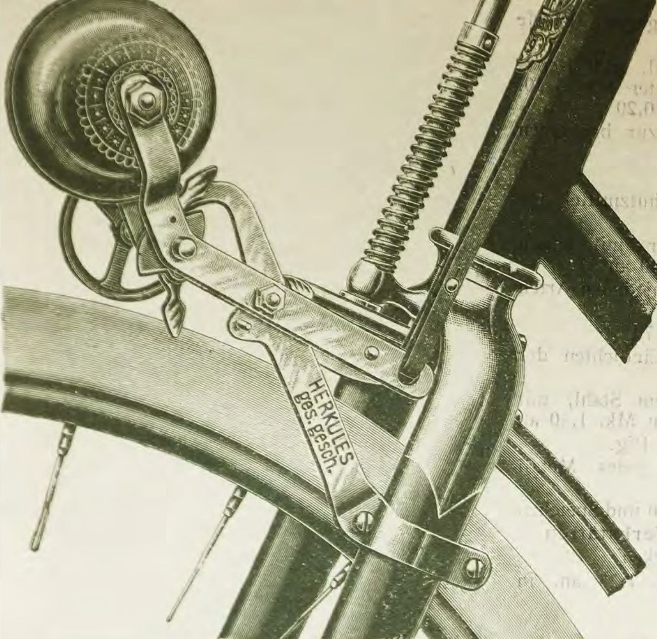
Nr. 884. Radläuferglocke „Herkules“ , kleines Modell.
