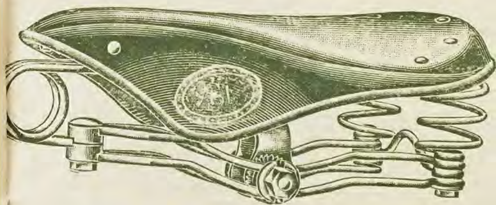
Nr. 82. Tourensattel mit doppelter Brücke. Best federnder Sattel für mittelschwere Fahrer, hochelegant. 27 cm lang, 19 cm breit. Gewicht 950 Gramm. Stück Mk. 3,25.
